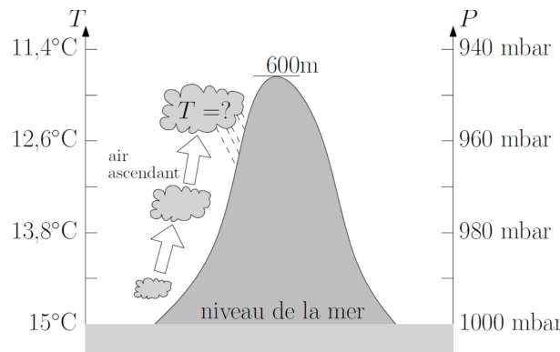
FIGURE 4 – Température et pression totale dans l'atmosphère
