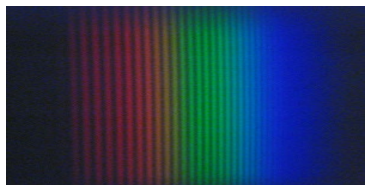
Spectre cannelé (blanc d'ordre supérieur)
