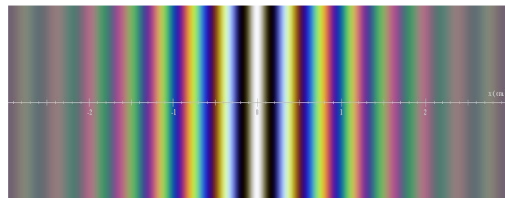
Eclairement dû aux différentes longueurs d'onde
