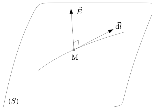
FIGURE 12 – Les lignes de champ sont perpendiculaires aux équipotentiels
