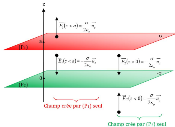
FIGURE 25 – Champ créé par un condensateur plan
