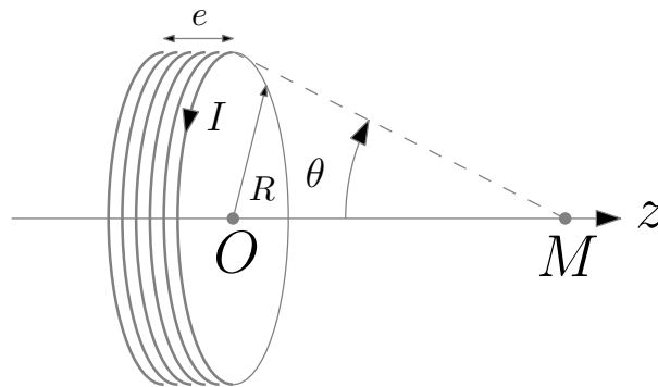
FIGURE 51 – Champ magnétique créé par une bobine
