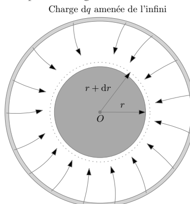
FIGURE 23 – Couche élémentaire amenée de l'infini
