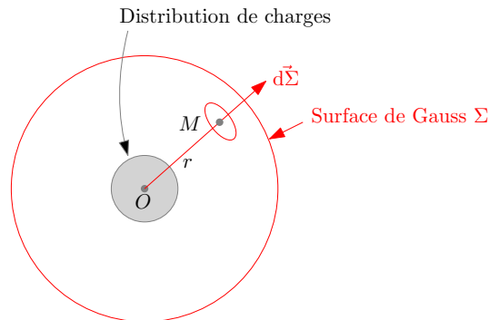
FIGURE 20 – Choix de la surface de Gauss
