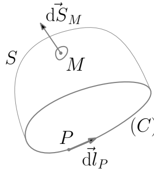
FIGURE 10 – Surface ouverte S et contour fermé orienté ( C )
