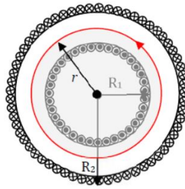
FIGURE 60 – Cas où M est à l'intérieur du tore
