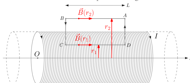
FIGURE 44 – Choix de la circulation
