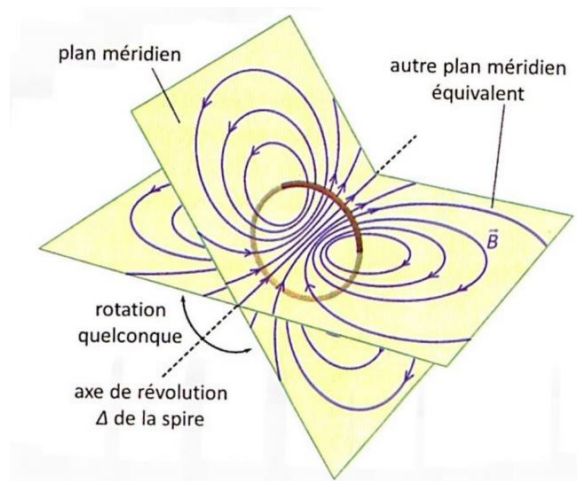
FIGURE 50 – Lignes de champ du champ magnétique crée par une spire
