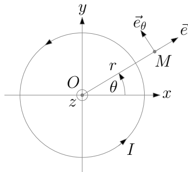
FIGURE 43 – Coordonnées cylindriques
