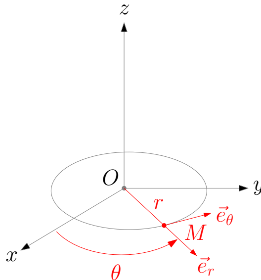
FIGURE 73 – Modèle de Bohr
