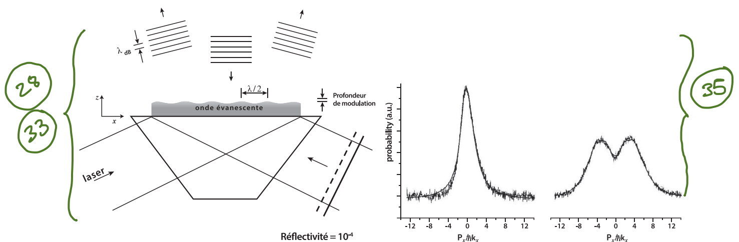
Figure 3: A gauche : Réseau de diffraction à atomes. Une petite fraction de la lumière incidente est renvoyée vers le prisme, créant une onde évanescente légèrement modulée. La profondeur des surfaces équipotentielles (amplitude verticale entre les sommets et les creux) est beaucoup plus petite que sa période. Une onde de de Broglie atomique subit une forte diffraction si \lambda_{dB} est de l'ordre de cette profondeur de modulation. Puisque \lambda_{dB} \approx \lambda/100 , les atomes sont sensibles à de très faibles déformations de l'onde évanescente. A droite : Mesure de la probabilité de diffraction atomique (en unité arbitraire) en fonction de la quantité de mouvement transverse P_x de l'atome en unité de \hbar k_x . La partie gauche correspond à la réflexion sur une surface plane. La partie droite représente la figure de diffraction sur un réseau de lumière pour lequel \varepsilon = 0,023 . Les pics correspondent aux deux premiers ordres diffractés (en \pm 2\hbar k_x et \pm 4\hbar k_x ) qui ne sont pas résolus.
